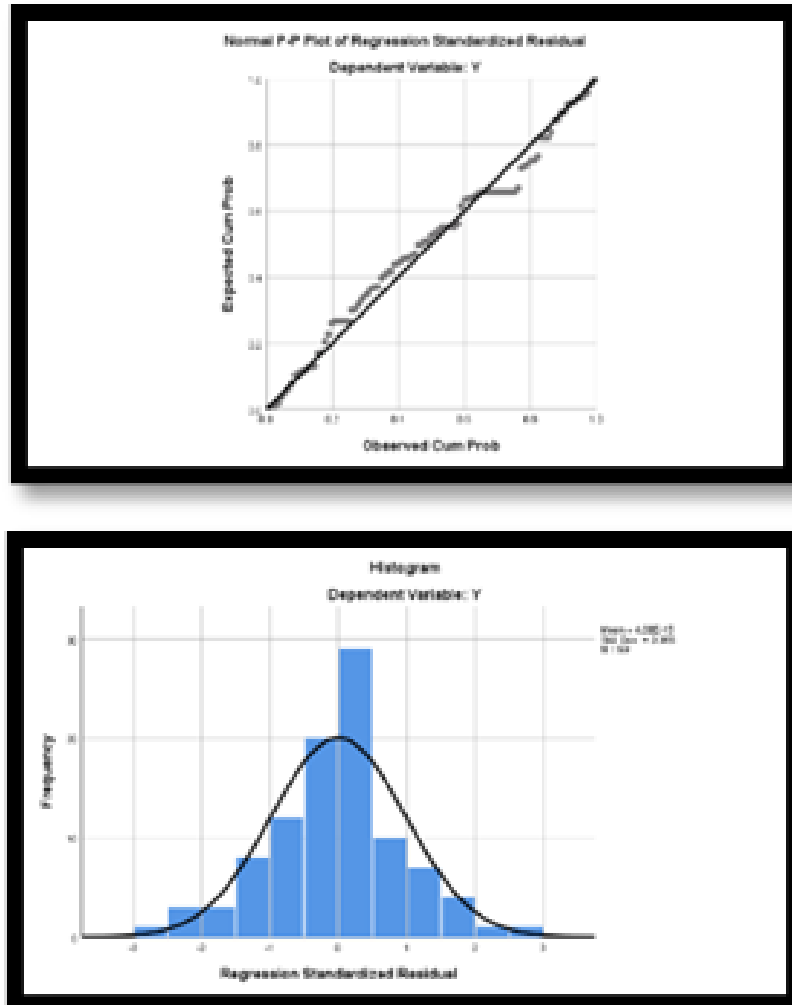
Gambar 1. Normal PP Plot dan Histogram
